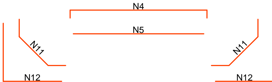
ARMAÇÃO CA-50 SEM ESCALA
