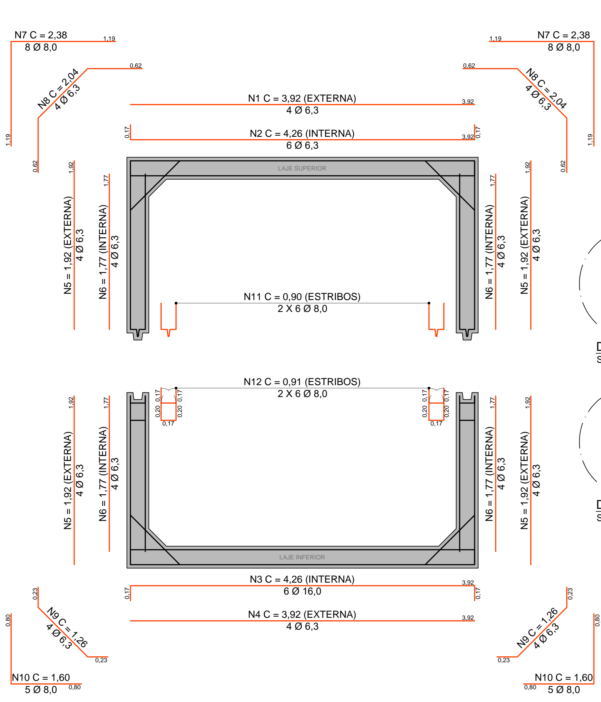
ARMAÇÃO AÇO CA-50 ESCALA 1:25
